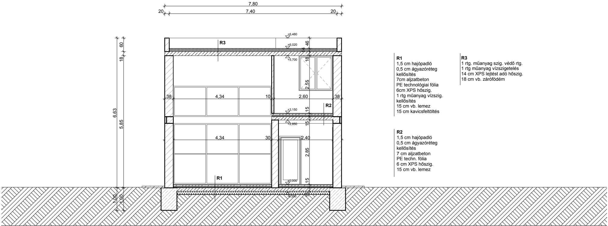
B-B metszet
