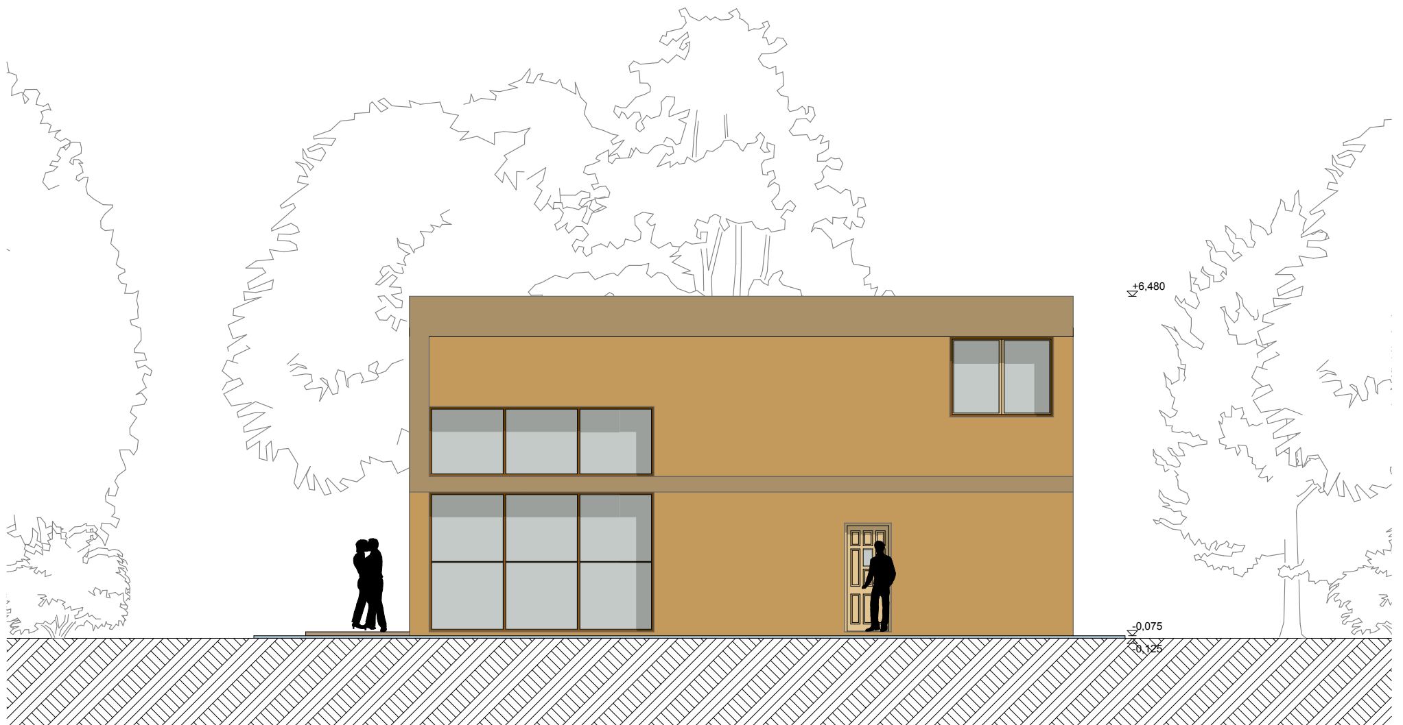
Déli homlokzat
