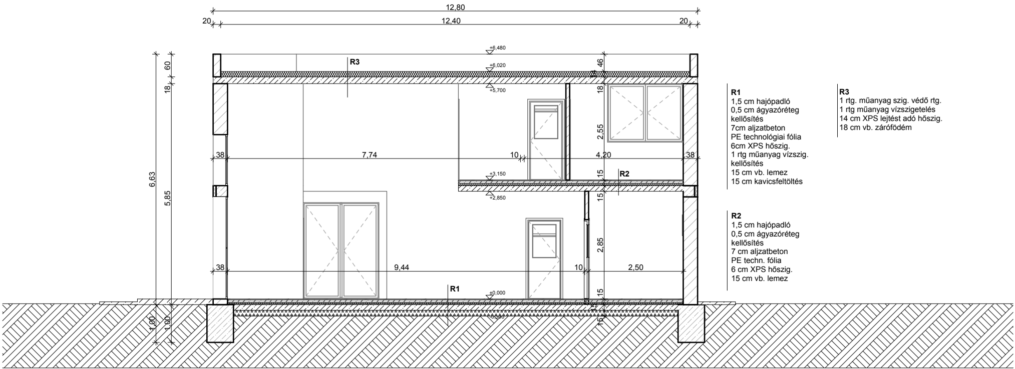
A-A metszet
