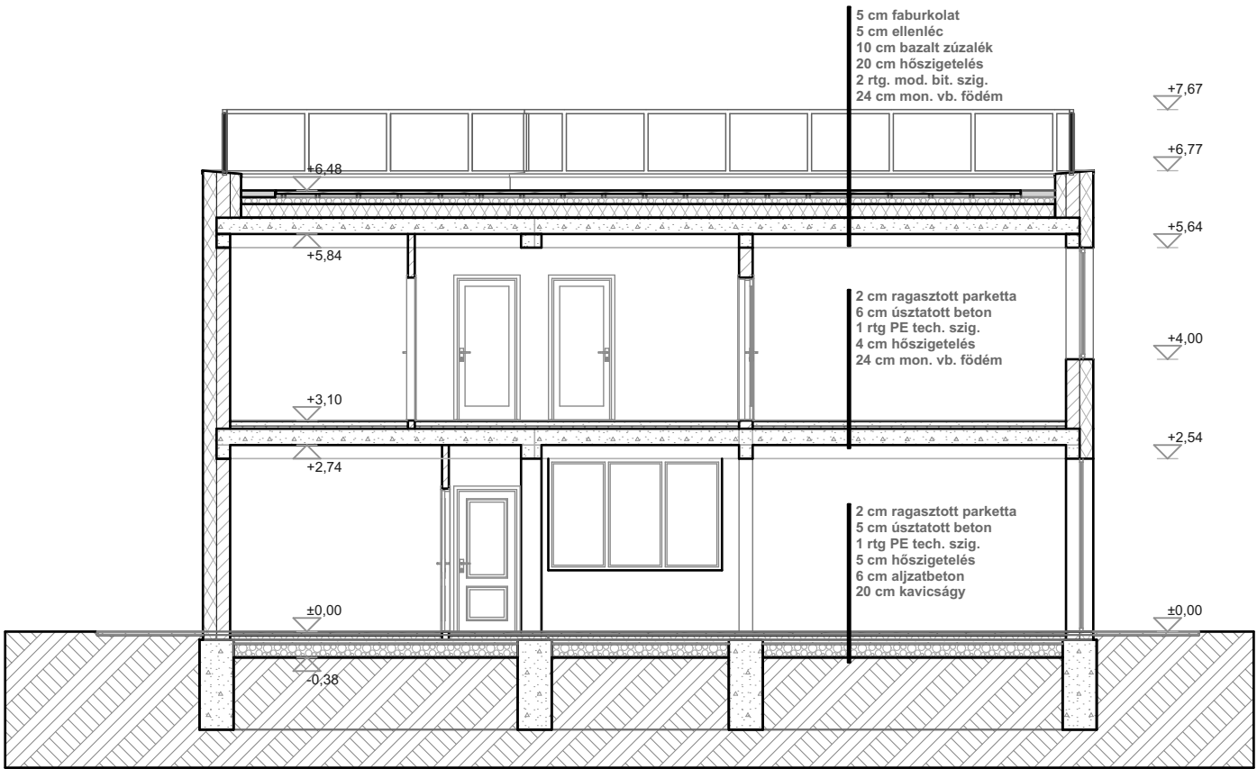
M-01 Metszet 1:100
