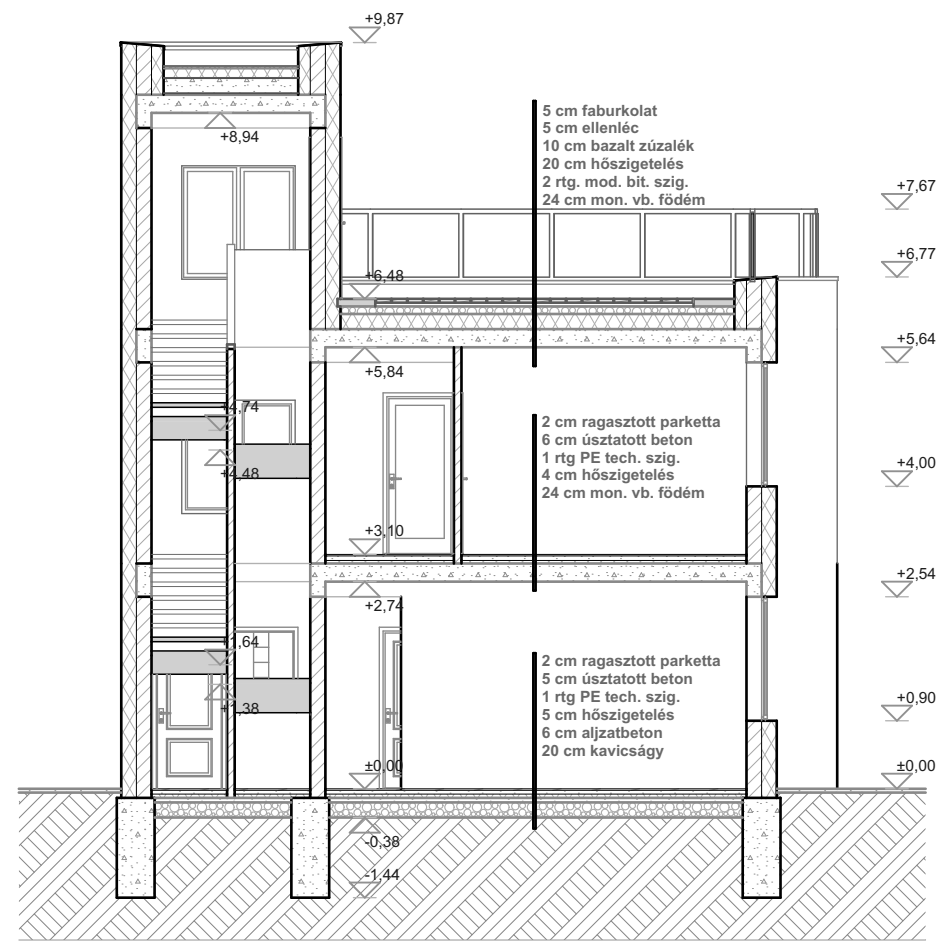
M-02 Metszet 1:100
